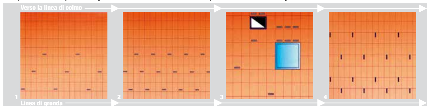
Fig.1 Per siti di altitudine inferiore a 750 mt. s.l.m (un elemento fermaneve ogni 5 elementi standard su tre file sfalsate in prossimità della linea di gronda). Per siti di altitudine tra 750 e 1200 mt. s.l.m (un elemento ogni 2 elementi standard, sempre su tre file). Fig.2 Per siti di altitudine tra 750 e 1200 mt. s.l.m (un elemento ogni 2 elementi standard, sempre su tre file).
